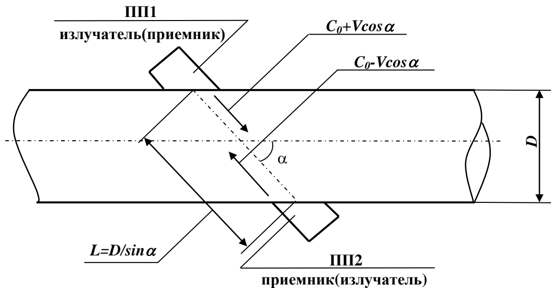
Рисунок 1 – Схема ИУ
